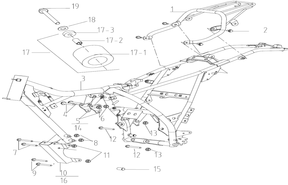
FIG.11 FRAME
