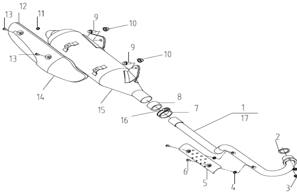
FIG.16 MUFFLER
